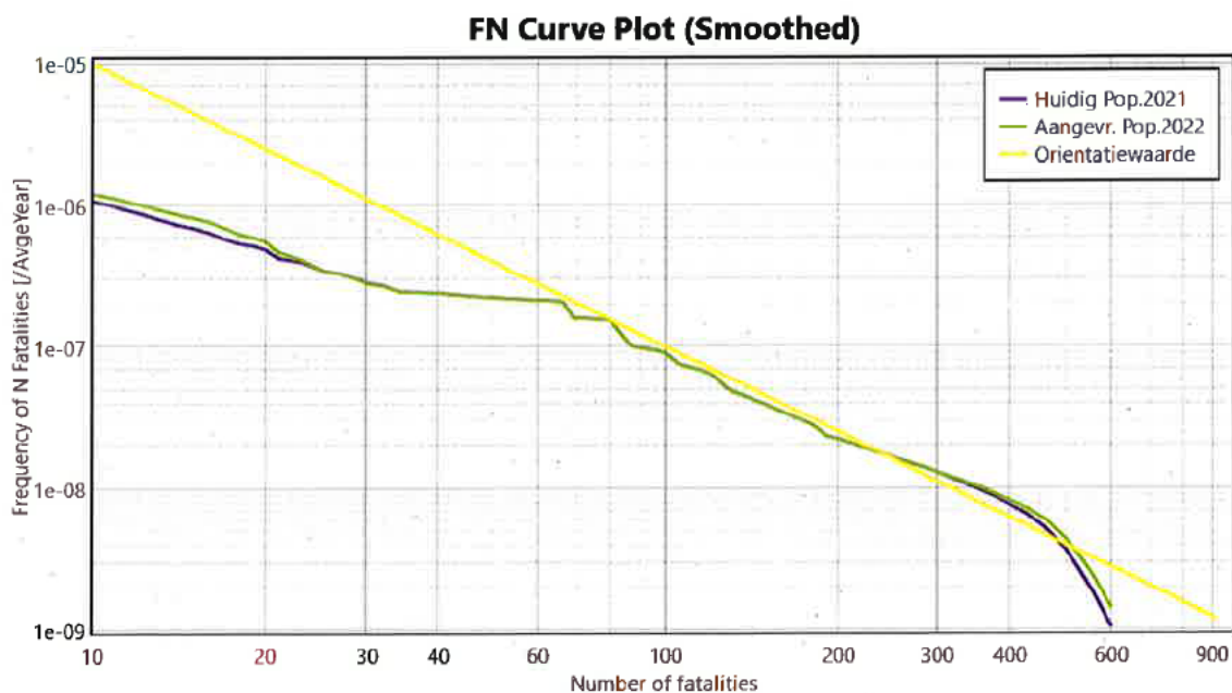
Figuur 2: Groepsrisico
