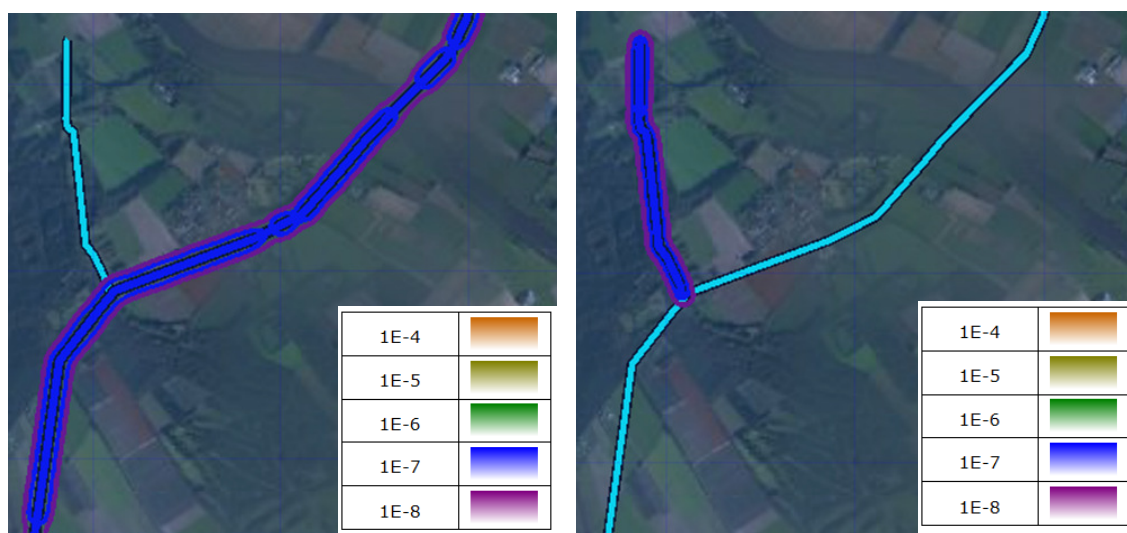
Figuur 20: resultaat PR berekeningen hogedruk aardgastransportleidingen Z-451-11( links) en Z-451-12( rechts)
