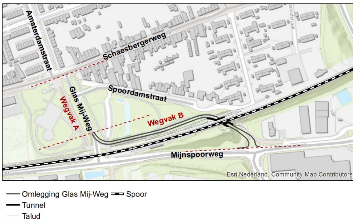
Figuur 6-1. Overzicht wegomlegging Glas Mij-weg. In wegvak A wordt de snelheid verlaagd naar 30 km/u. Wegvak B is de nieuwe aanleg.
